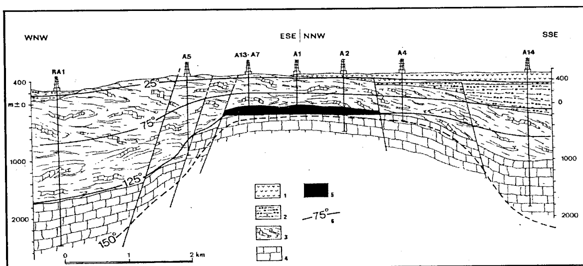
1) vulcaniti - 2) depositi marini pliocenici - 3) facies ligure ed austrapina interna - 4) facies toscana - 5) cappa di gas - 6 isoterme Campo geotermico di Torre Alfina - Schematica su una traccia in corrispondenza dei Pozzi Enel
